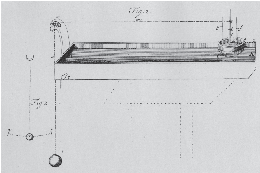
4. Experimentmaskin för provande av skeppsmodeller. Emanuel Swedenborg, Prodromus principiorum rerum naturalium sive novorum tentaminum chymiam et physicam experimentalem geometrice explicandi (1721).
