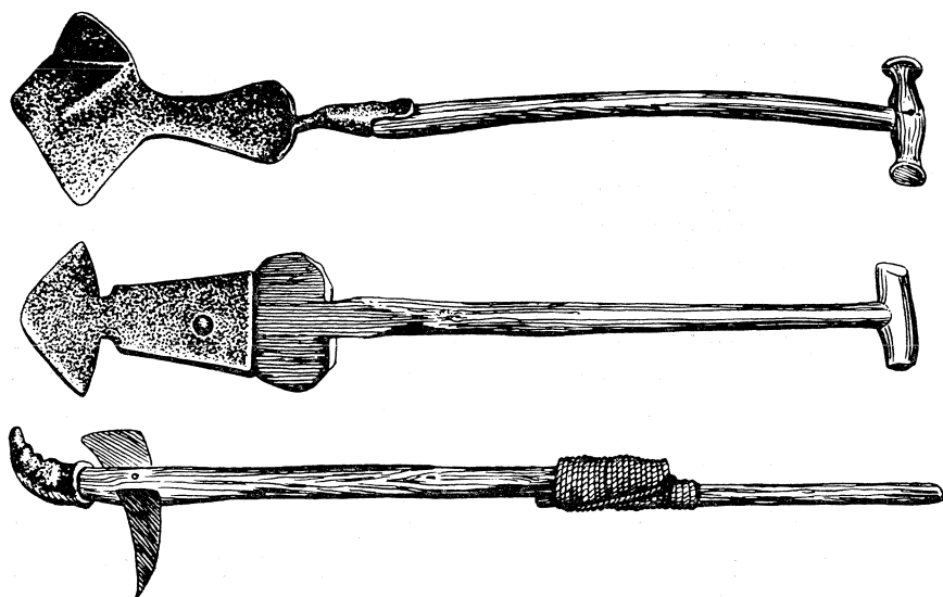
Fig. 5—7. Torvspadar och torvriv från Darum, Ulsted respektive Fanö. Landbrugsmuseet nr 4603, 4594, 4659. Skala 1 : 10.
