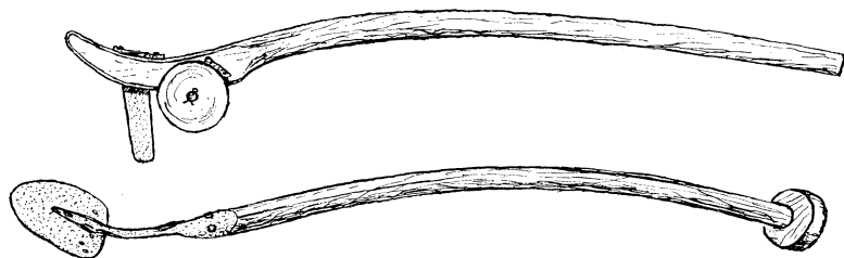
Fig. 11—12. Redskap för upptagning av »torvsvär» från Ö. Tommarp. Österlens museum nr 2771, 4091: A. Jfr även 2146 från Simris. Skala 1 : 15.
