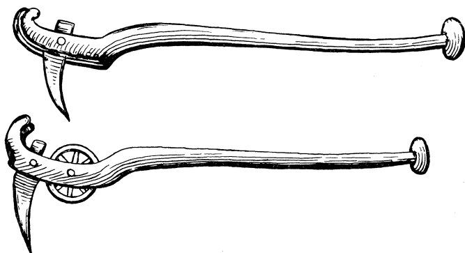
Fig. 13—14. Ristar för dikesupptagning. Efter W. Blith, The English Improver Improved .
