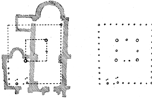
Abb. 1. Die gefundenen Pfostenlöcher unter der früheren Domkirche zu Alt-Uppsala (nach Lindqvist 1926) und eine Rekonstruktion der beiden Pfostenloch-Vierecke.
