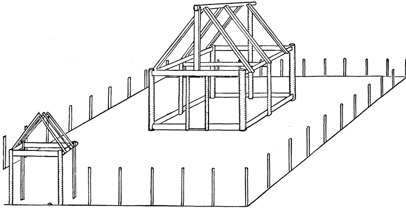
Abb. 2. Versuch einer holzbautechnischen Rekonstruktion vom Gerüst des Uppsalatempels, mit Einfriedigung.
