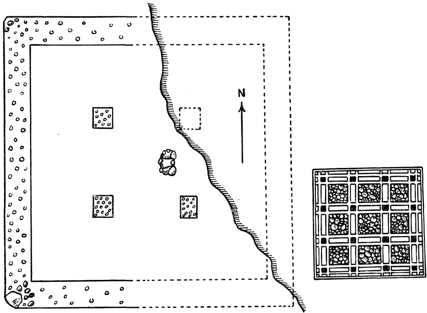
Abb. 4. Die Grundrisse von dem Tempel Arkona (nach Schuchhardt 1921) und dem Glockenturm Häverö (nach M. Olsson 1912) in demselben Massstab.
