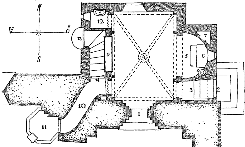
PLAN AV SÖNDRUMS SAKRISTIA I SKALA 1/100.
