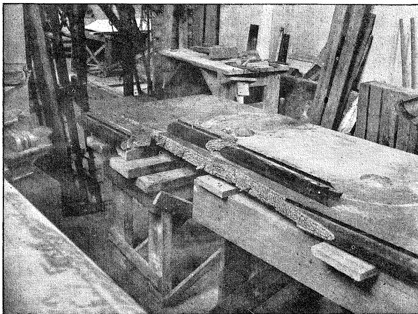
FIG. 10. LOCKETS ÖVERSTYCKE UNDER PÅGÅENDE LAGNINGARBETE. I BROTTYTAN INBORRADE BRONSDUBBAR FÖR VILKA FINNAS MOTSVARANDE HÅL I DE OVANFÅ SKIVAN LIGGANDE LÖSA BITARNA.
