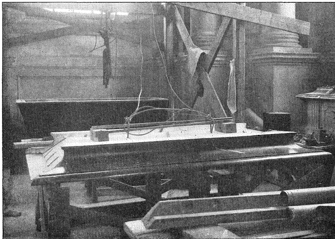
FIG. 12. LOCKETS LÅNGSIDOR UPPMONTERAS EFTER SAMMANFOGNINGEN PÅ DEN BÄRANDE BETONGSTOMMEN. I BAKGRUNDEN SARKOFAGENS FÄRDIGRESTAURERADE UNDERDEL.
