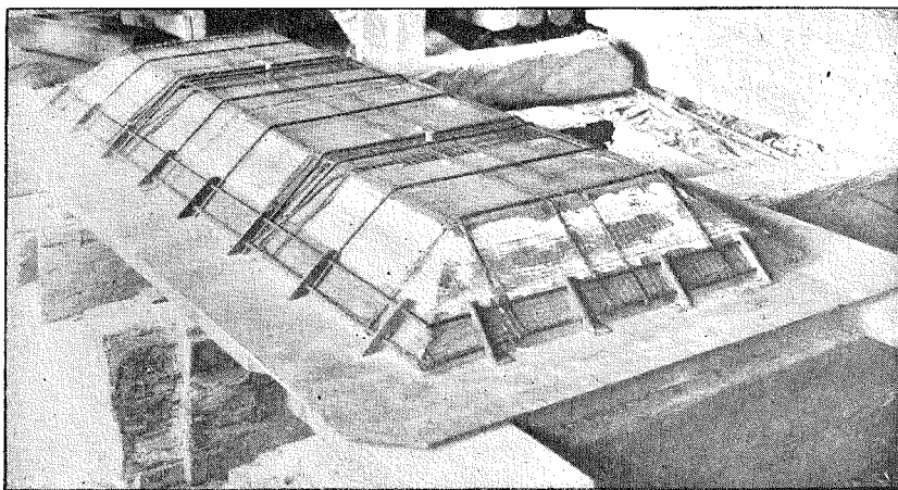
FIG. 9. BRONSRAMEN OCH JÄRNSKELETTET TILL LOCKETS CEMENTSTOMME UPPMONTERADE PÅ TRÄMODELLEN FÖRE GJUTNINGENS BÖRJAN.
