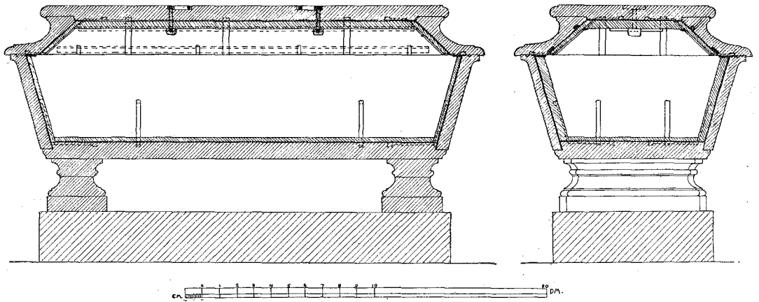
FIG. 3. SARKOFAGENS LÄNGD- OCH TVÄRSEKTIONER FÖRE RESTAURERINGEN.
