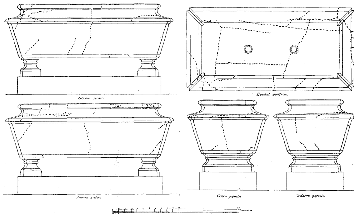
FIG. 2. UPPMÄTNINGSRITNING AV SARKOFAGEN VISANDE DE FÖRE DESS ÖPPNANDE SYNLIGA SPRICKORNA.
