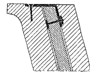
FIG. 6. DETALJ AV FIG. 4 VISANDE DE YTTRE MARMORSKIVORNAS FÄSTANDE VID DEN BÄRANDE STOMMEN.
