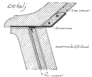
FIG. 5. DETALJ AV FIG. 4 VISANDE KONSTRUKTIONEN AV LOCKETS BÄRANDE STOMME.
