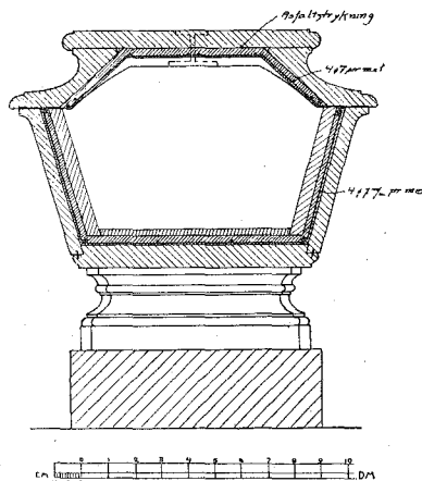
FIG. 4. SARKOFAGEN SEDD I TVÄRGENOMSKÄRNING EFTER RESTAURERINGEN.
