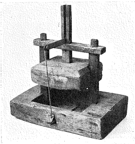
Fig. 9. Rättfälla med klumpkonstruktion. Näs socken, Dalarna. Nordiska museet.
