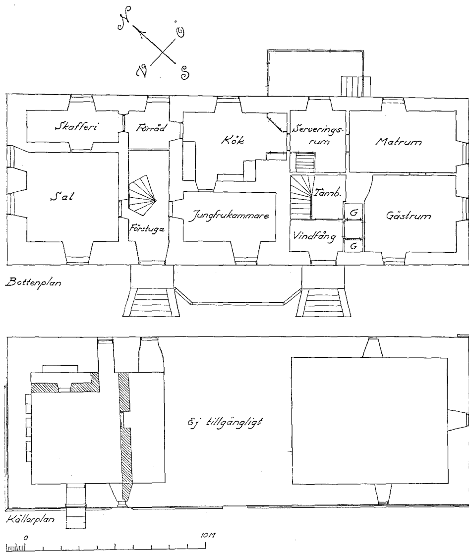
Fig. 4—5. Planer av botten- och källarvåningarna före restaureringen 1936. Sekundära mellanväggar i källaren skrafferade. Skala 1: 200.
