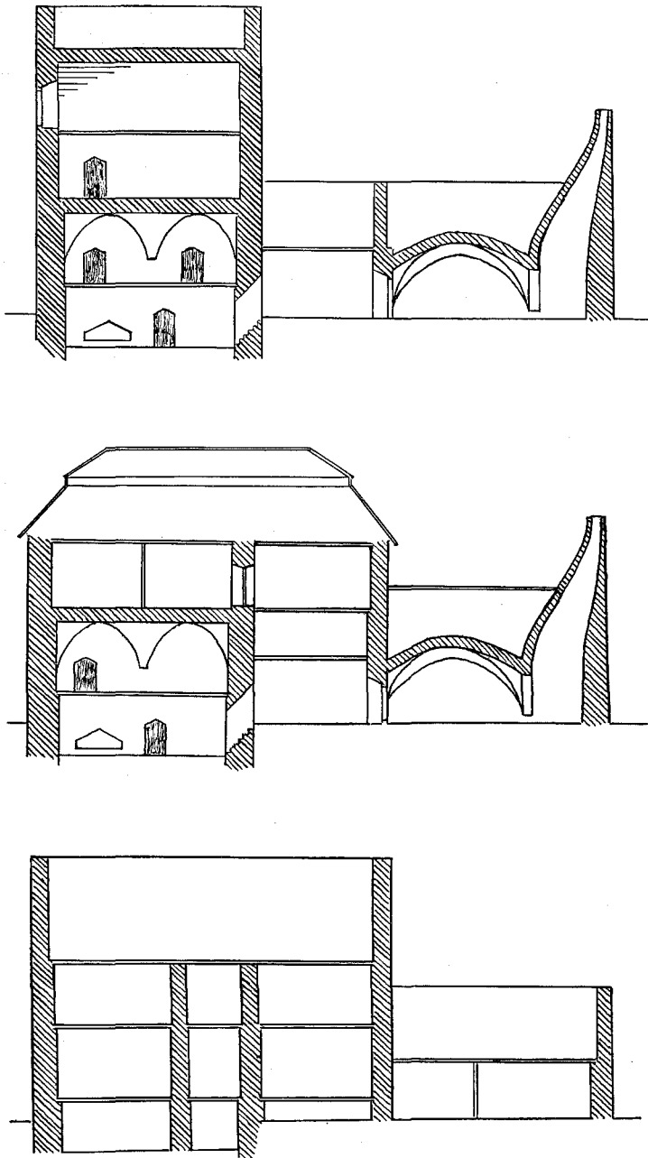
Fig. 8—10. Schematiskt rekonstruerade sektioner av byggnaden vid olika tider. Överst vid 1200-talets slut, därunder vid husesynen 1749, underst efter ombyggnaden på 1760-talet. Skala 1: 300.
