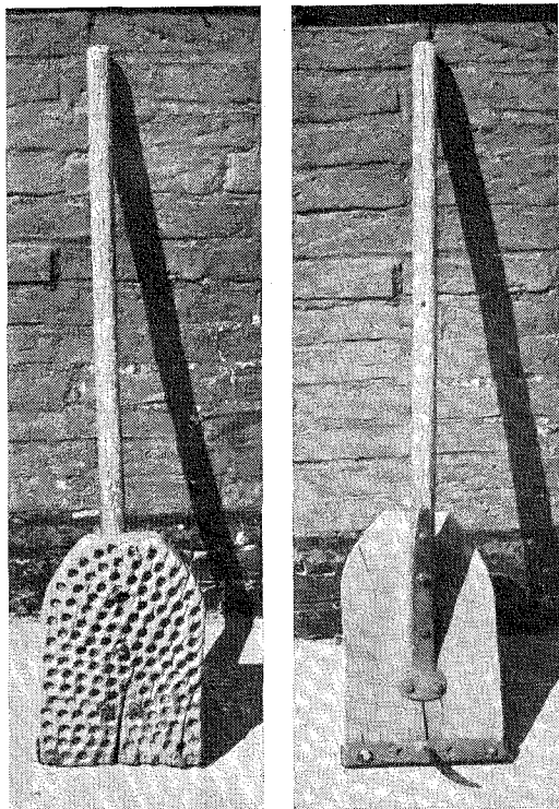
13. Täckeskovel från Mjølby, Rømø sn, Højer hd, Jylland. Total längd 1,90 m, bladet 32×19 cm. Nationalmuseet, Köpenhamn.
