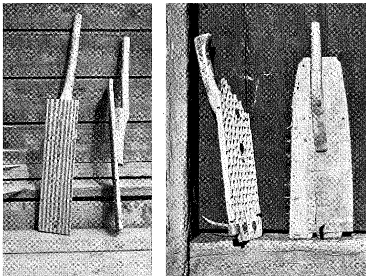
5 a. Räfflade vrakor från Lahlolms sn, Höks hd, Halland. 98×8×1½ cm resp. 41×10×1,3 cm. Obs.! de relativt långa skaften. b. Hålade vrakor från Harplinge sn, Halmstads hd, Halland. Foto förf.
