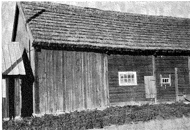
11. Tak av vass ("bla-rö"). Bläsinge, Högbo sn, Åkerbo hd, Öland. Obs.! skiktningen på taket, lagt 1948.
