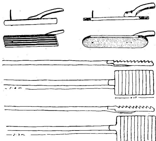
12 a-b. Täckevrakar från Danmark. Efter Nationalmuseets etnologiske undersøgelser: spørgeliste nr 3. c-d (nedre figurerna). Äldre täckevrakar från Vorumaa, Estland. Efter Manninen.
