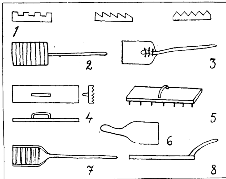
10. Täckevrakor (efter meddelarnas teckningar eller beskrivningar).
