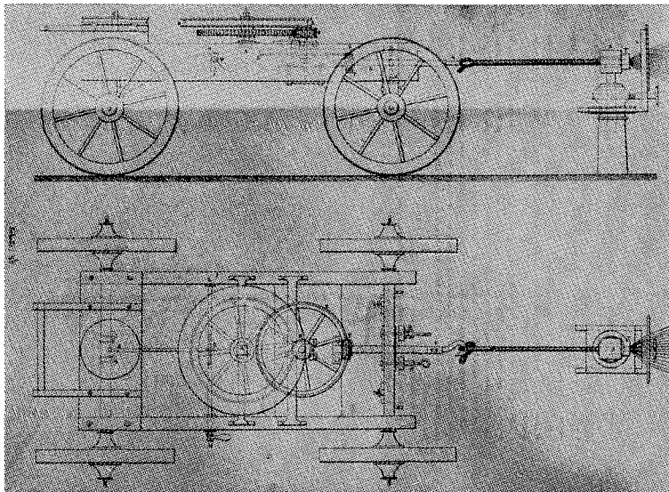
4. Dragvagn med drivhjul från Toulon. Ur M.A.L. Chédévilles arbete, Paris 1839.
