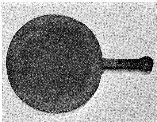
4. Stenkaksjärn från Urshult, Kinnevalds härad. Nordiska museet nr 238.201. Diam. 30 cm, total längd 45 cm, tjocklek 1 cm, vikt 6200 gr. Det mörkare partiet på järnet visar stenkakans omfång.
