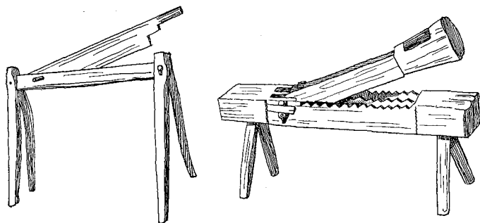
1. Linbråka. Csongrád, Ungern. Efter Szolnoky 1966. 2. Linbråka. Jászapáti, Ungern. Efter Szolnoky 1966.
