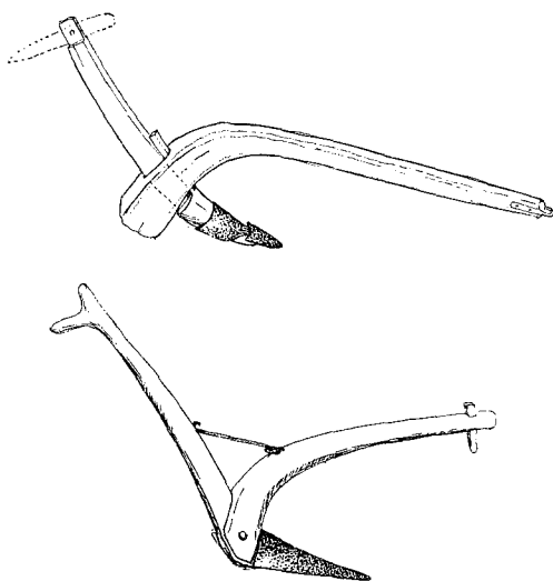
4. Överst: Ard, Svegs sn, Härjedalen. Nederst: Ard, Hanebo sn, Hälsingland. Foto etter Svensk Geografisk Arsbok, 1949, s. 150, 151 (Sigurd Erixon).
