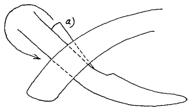
5. Skjematisk tegning av ard med "hullfeste". Kilen a) kan flyttes ned under ardbuen og endre vinkelen mellom dragåsen og ardbuen.
