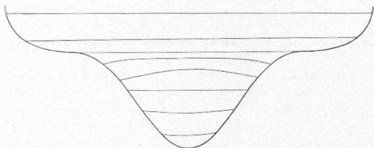
Fig. 4. Diagramm über die O_2 -Schichtung im Skärhultssee. Die horizontale Sprungschicht, deren Lage von der allgemeinen Tiefe des Sees bestimmt wird, ist durch zwei horizontale Linien zunächst der Oberfläche angegeben. Darunter kommt eine Schichtung, nur wenig von der Bodenkonfiguration bestimmt.
